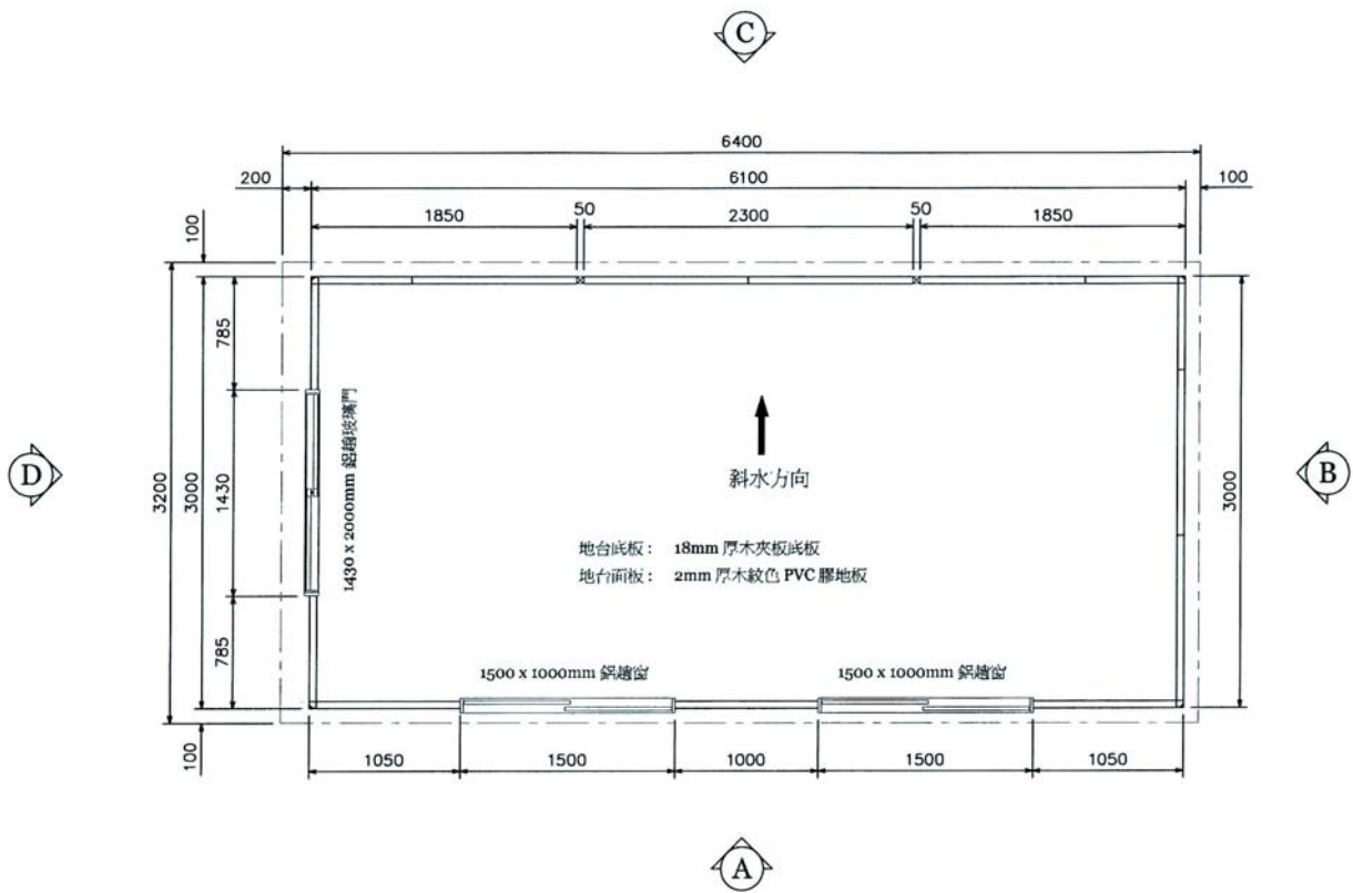
平面圖
